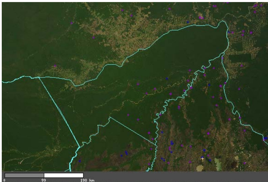
DISTRIBUCIÓN DE FOCOS DE CALOR DEL DEPARTAMENTO CON IMAGEN MODIS DE FECHA 06-OCT-2010
