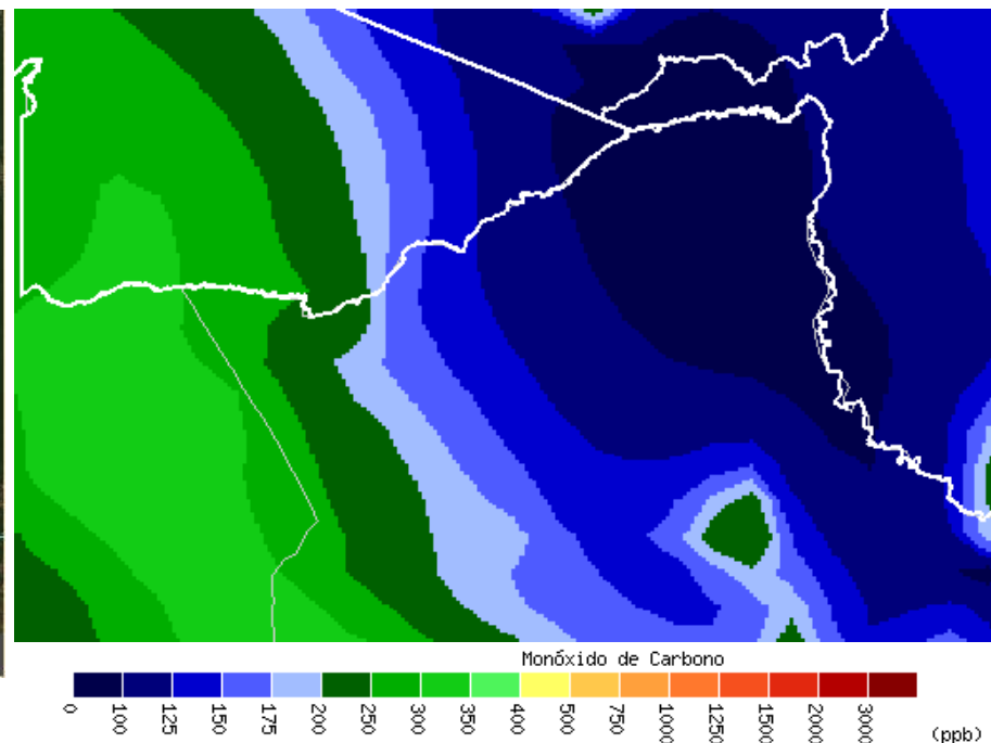
DISTRIBUCIÓN DEL MONÓXIDO DE CARBONO EN LA REGIÓN DE FECHA 06-OCT-2010
